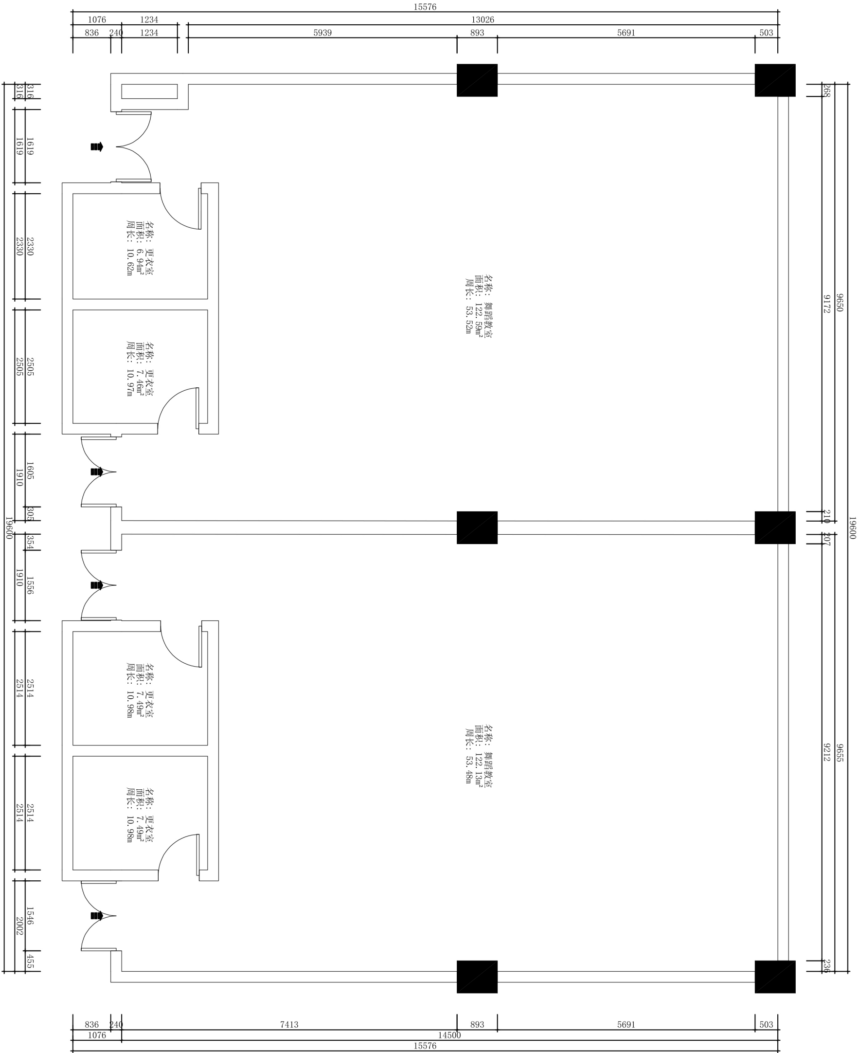
原始户型图
