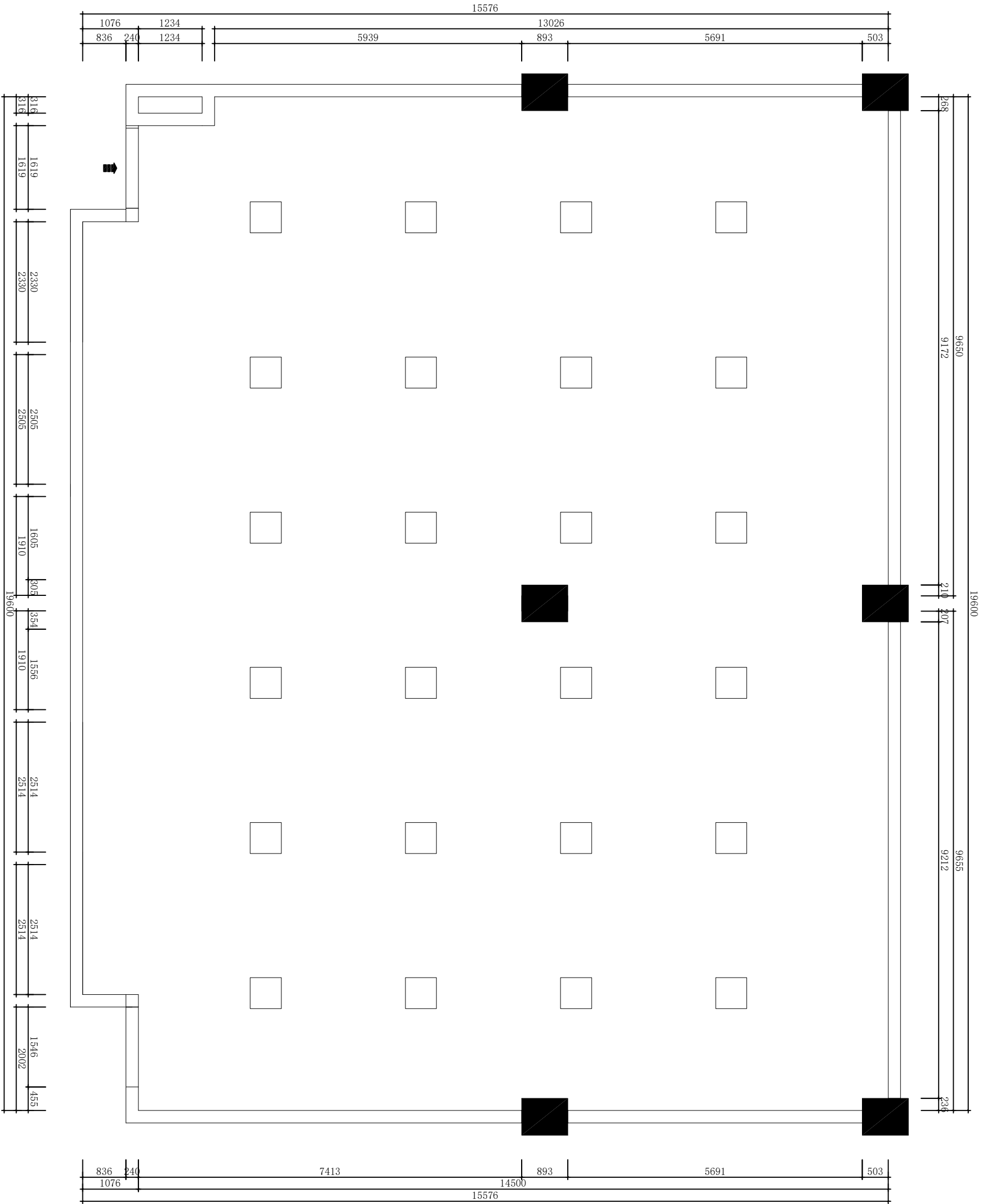
顶面布置图
